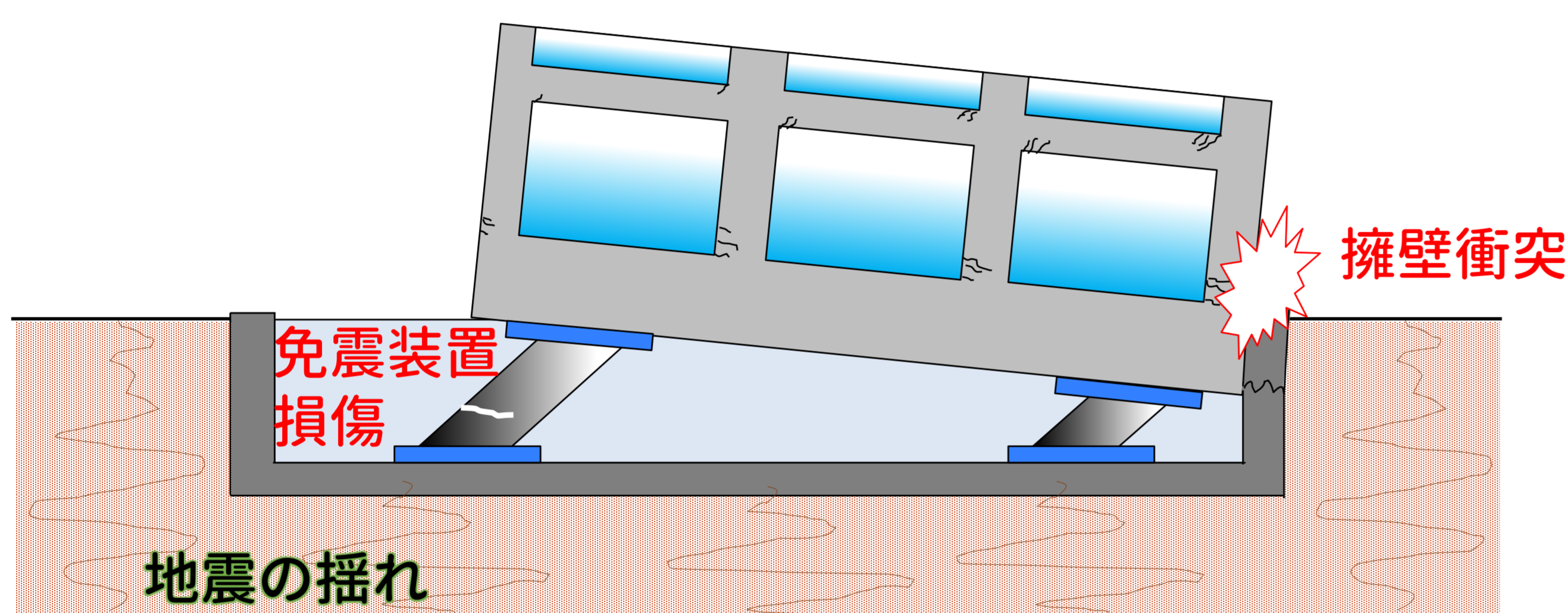
巨大地震を考慮しない免震構造で懸念される状況
