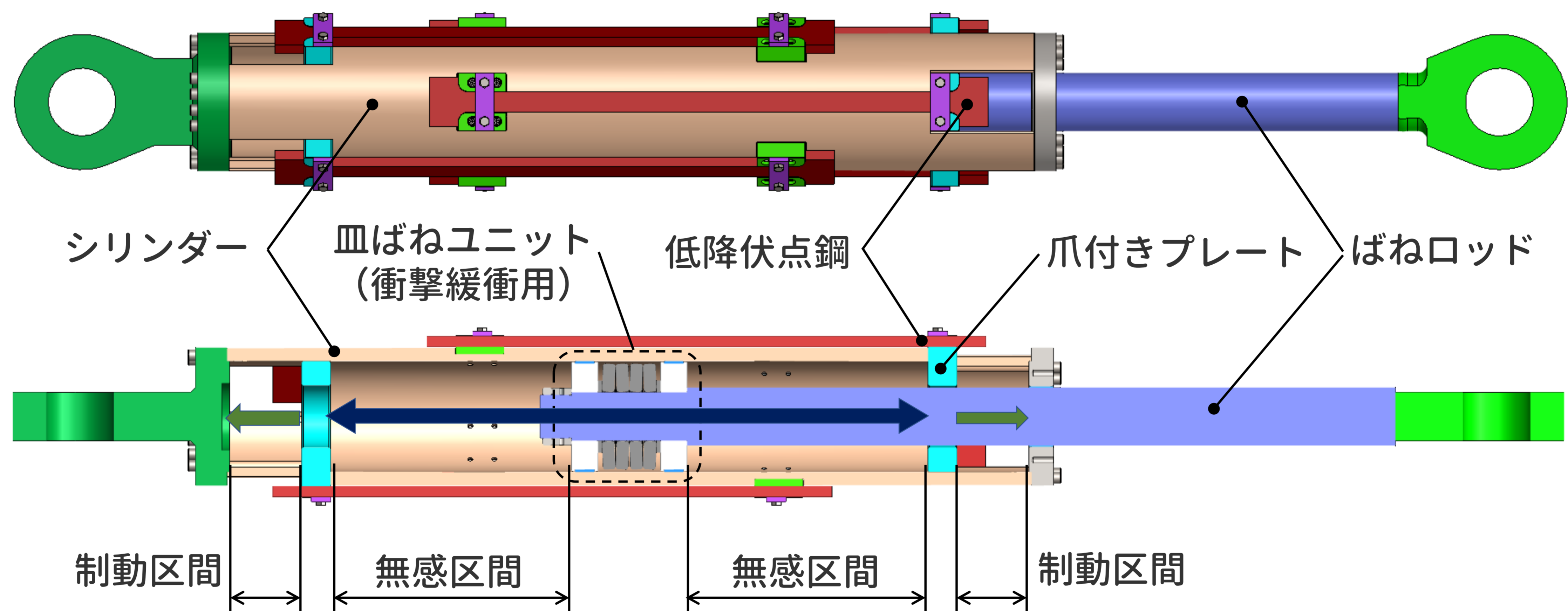
フェイルセーフ制動装置
