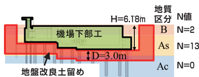
(b) 断面図
