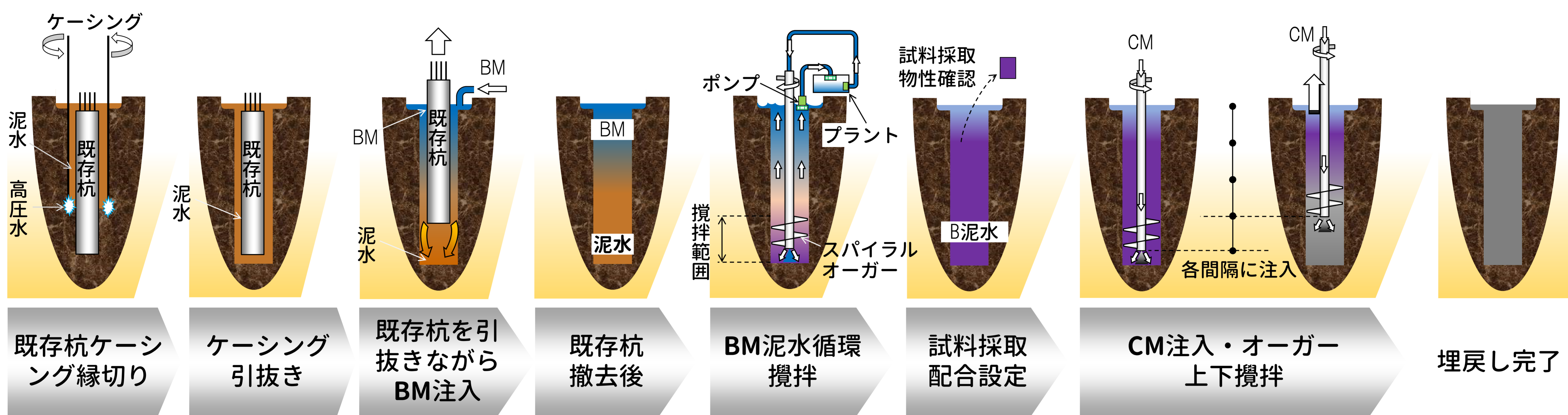
循環攪拌を用いたケーシング縁切り引抜き工法
