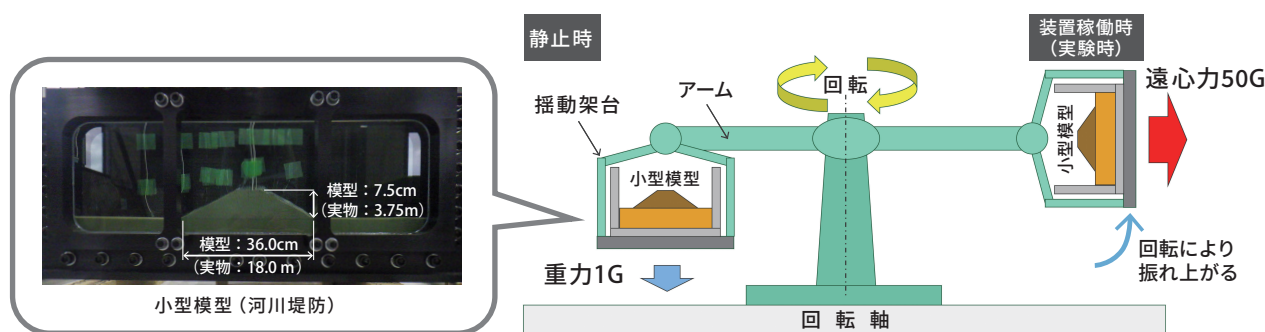
遠心力載荷装置概要図
