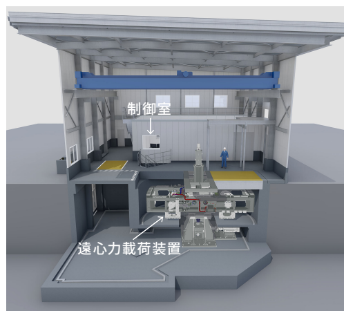
遠心載荷実験棟パース図
