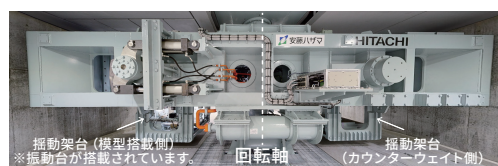
遠心力載荷装置
