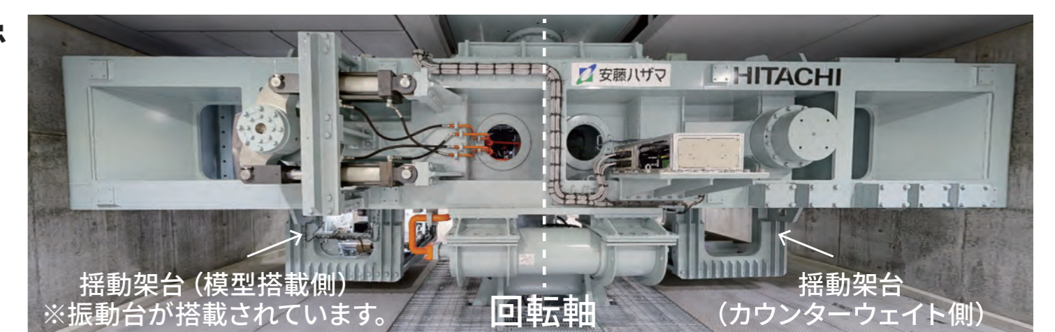
遠心力荷重装置
